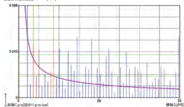
谐波分析结果[圆度<Round_15>]
